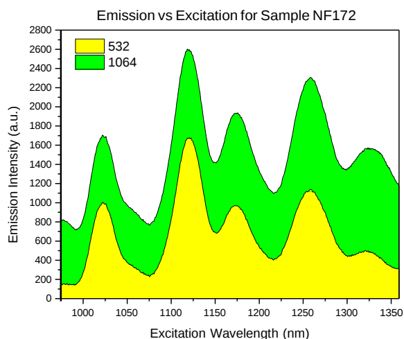
ΔΙΑΓΡΑΜΜΑ 1: Ένταση ακτινοβολίας εκπομπής και διέγερσης σαν συνάρτηση του μήκους κύματος
